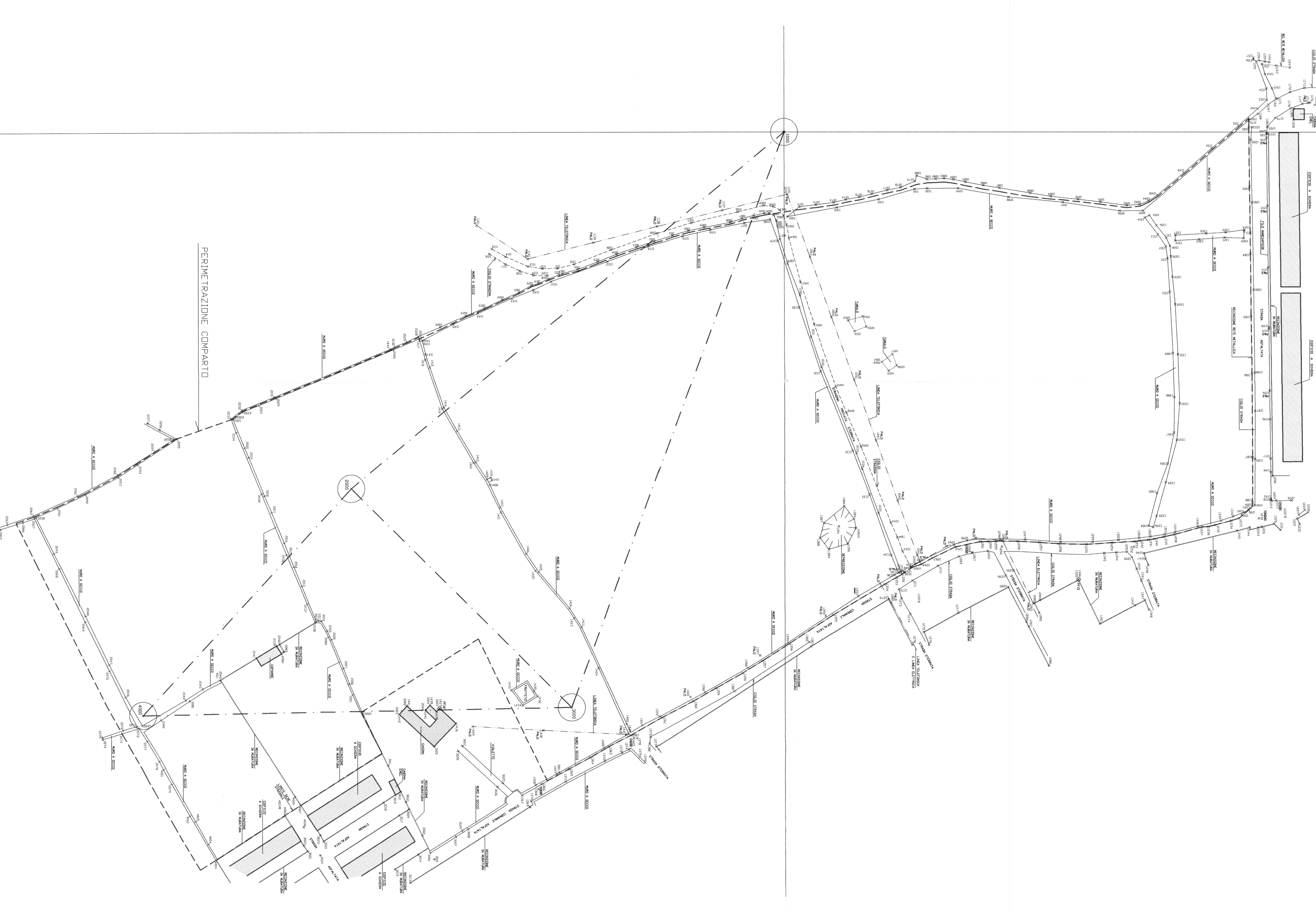
RILIEVO CELERIMETRICO DELLO STATO DEI LUOGHI - rapp. 1:1.000
